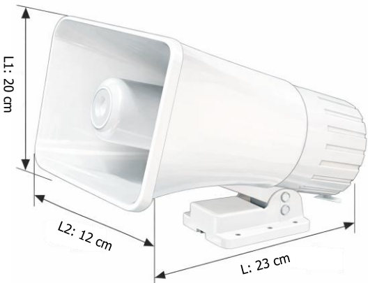
L1: altura de la boca de la bocina, L2: ancho de la boca de la bocina, L: largo total del equipo
